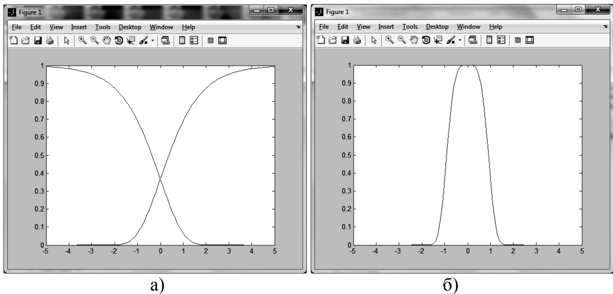
Рис. 25 – Приклади графіків функцій Харінгтона, де: а – для односторонніх обмежень, б – для двосторонніх обмежень
