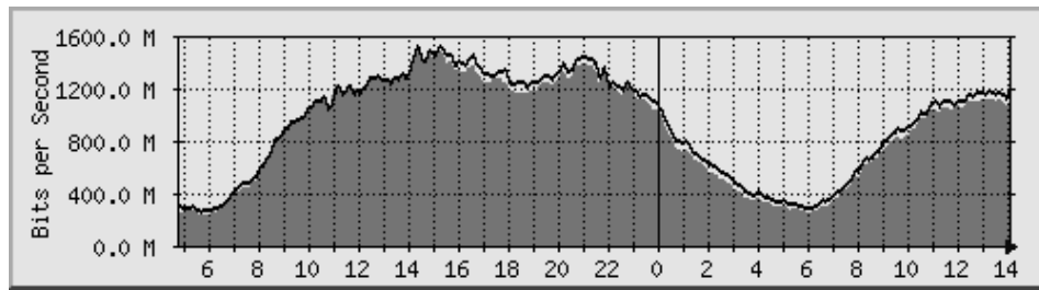
Рис. 3 – Добовий графік завантаження провайдера Israel Internet Exchange [17]
