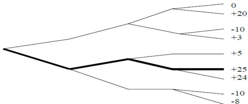
Рис. 14.10. Дерево рішень
