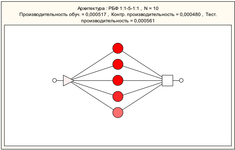
Рис.6.10. Архітектура нейромережевої моделі динамічного ряду UB ,
