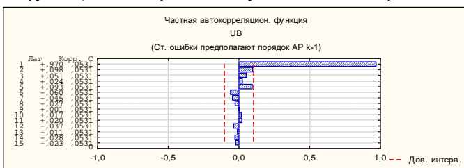
Рис.3.11. Графік та значення ЧАКФ динаміки UB, .
