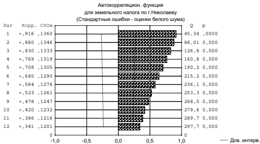
Рис.3.7. Автокорреляційна функція для земельного податку по м. Николаїв
