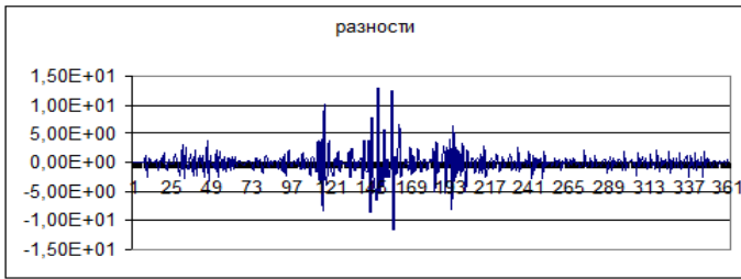
Рис.3.15. Графік третіх кінцевих різниць
