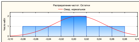
Рис.4.3. Діаграма нормального розподілу залишків моделі.
