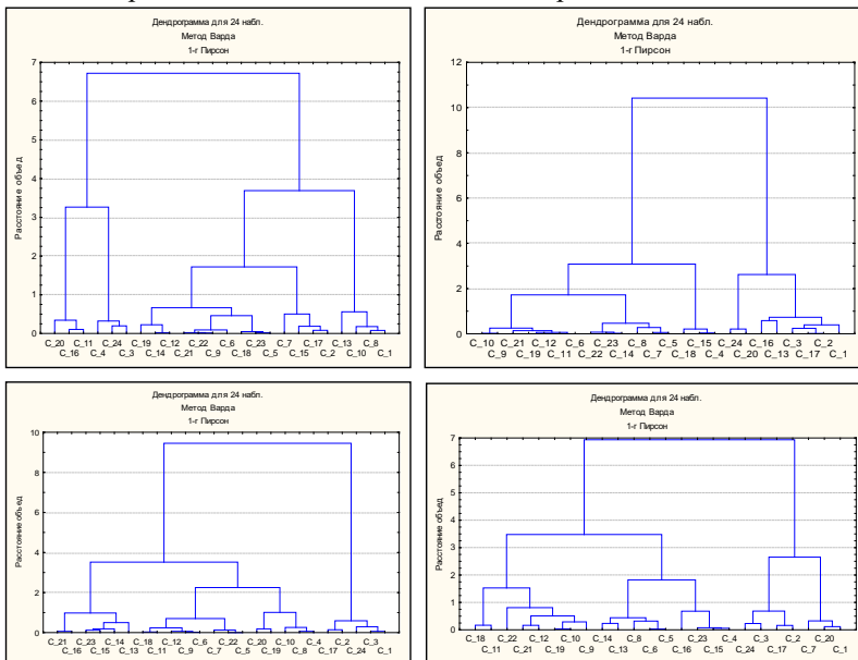
Рис. 2.7. Дендродіаграми розподілу підприємств на кластери за результатами їх діяльності (за результативними показниками y_j, j = \overline{31,36} ) протягом 2008-2011 років.
