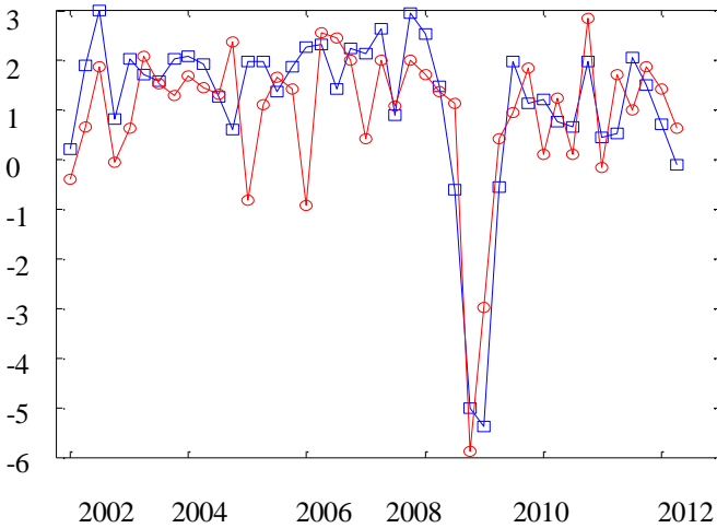
Рис.3.17. Фактичні (квадрати) та прогнози (круги) значення росту реального ВВП РФ, в % до попереднього кварталу з корегуванням на сезонність. Прогноз – на основі інформації за станом на кінець третього місяця відповідного кварталу. Прогнозна модель - DFM із трьома факторами. Горизонт прогнозування – поточний квартал.
