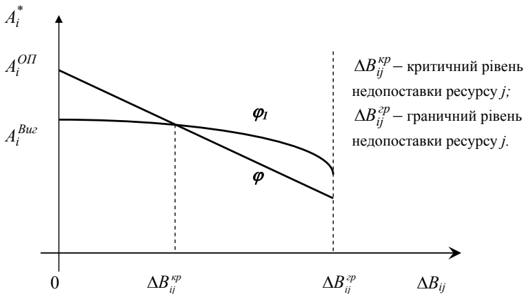
Рис. 6.16. Схема взаємозв'язку випуску продукції і недопоставки ресурсів
