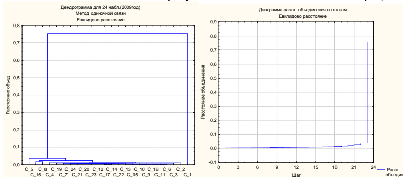
Рис. 2.6. Дендрограма ієрархічної класифікації та графік схеми об'єднання.
