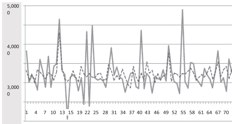
Рис. 6.12. Відтворення відносних змін надходжень ПДВ за регіонами по першому кварталу із застосуванням лінійної моделі
