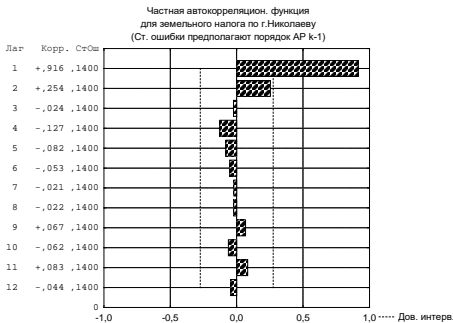
Рис.3.8. Частинна автокорреляційна функція для земельного податку
