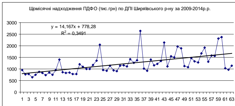
Рис.3.4. Динаміка щомісячних надходжень ПДФО (тис.грн) по Ширяївській ДПП за 2009-2014 роки.
