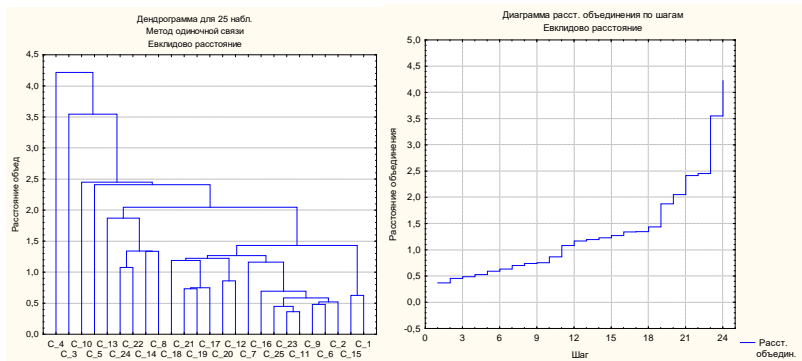
Рис. 2.5. Дендрограма ієрархічної класифікації та графік схеми об'єднання.
