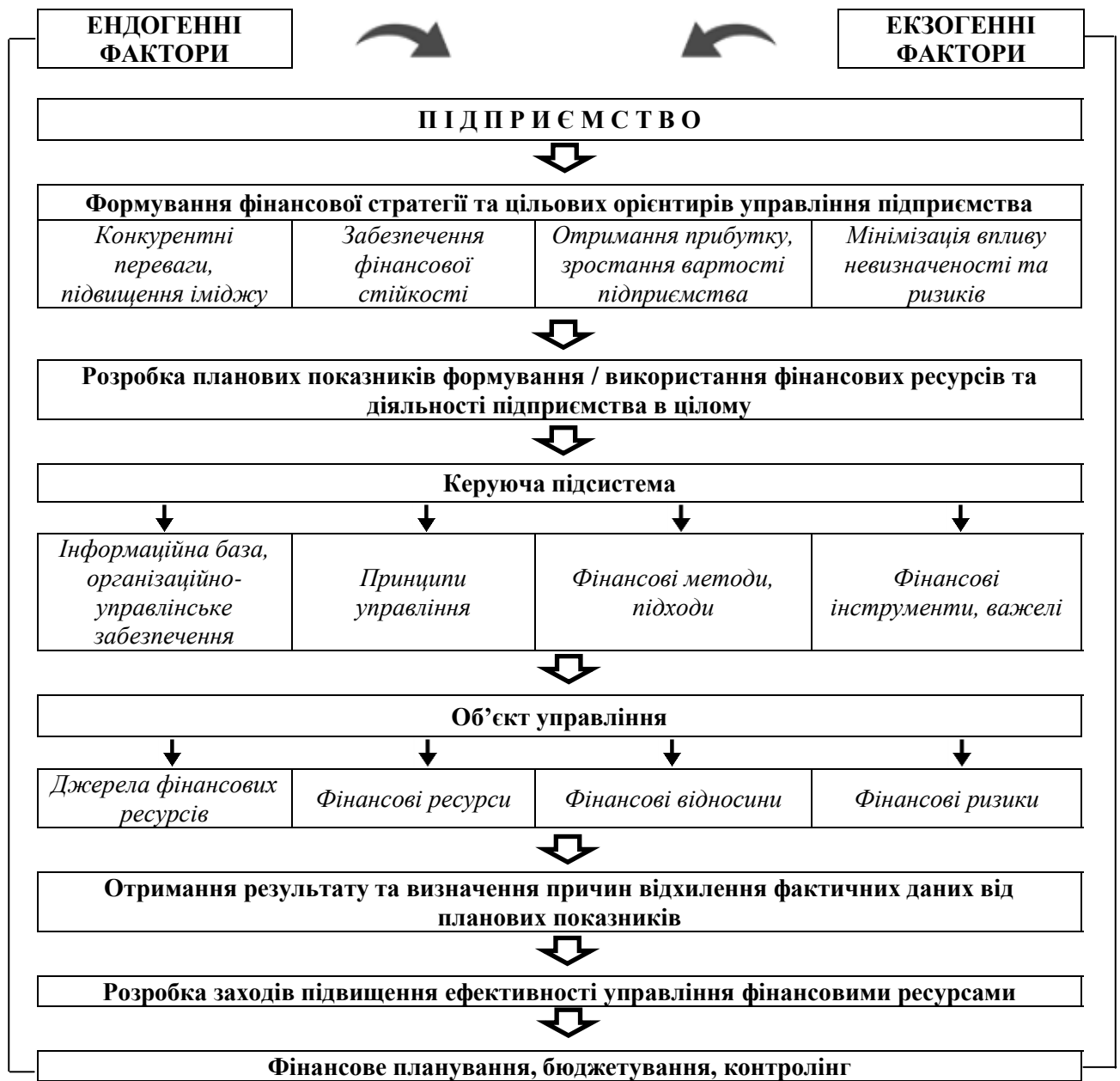
Рис. 2. Модель оптимізації управління фінансовими ресурсами промислового підприємства
