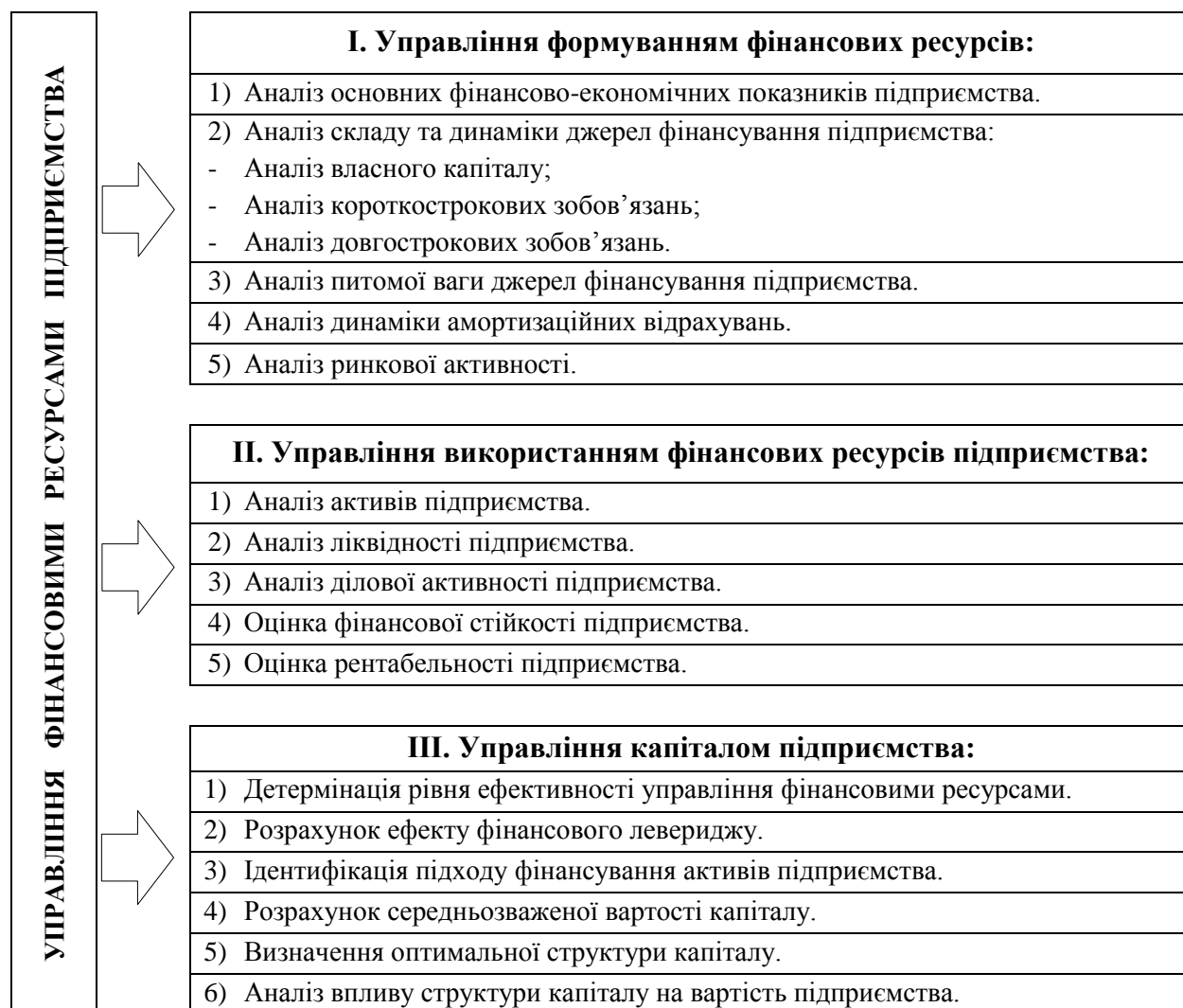
Рис. 1. Алгоритм аналітичного оцінювання управління фінансовими ресурсами промислового підприємства
