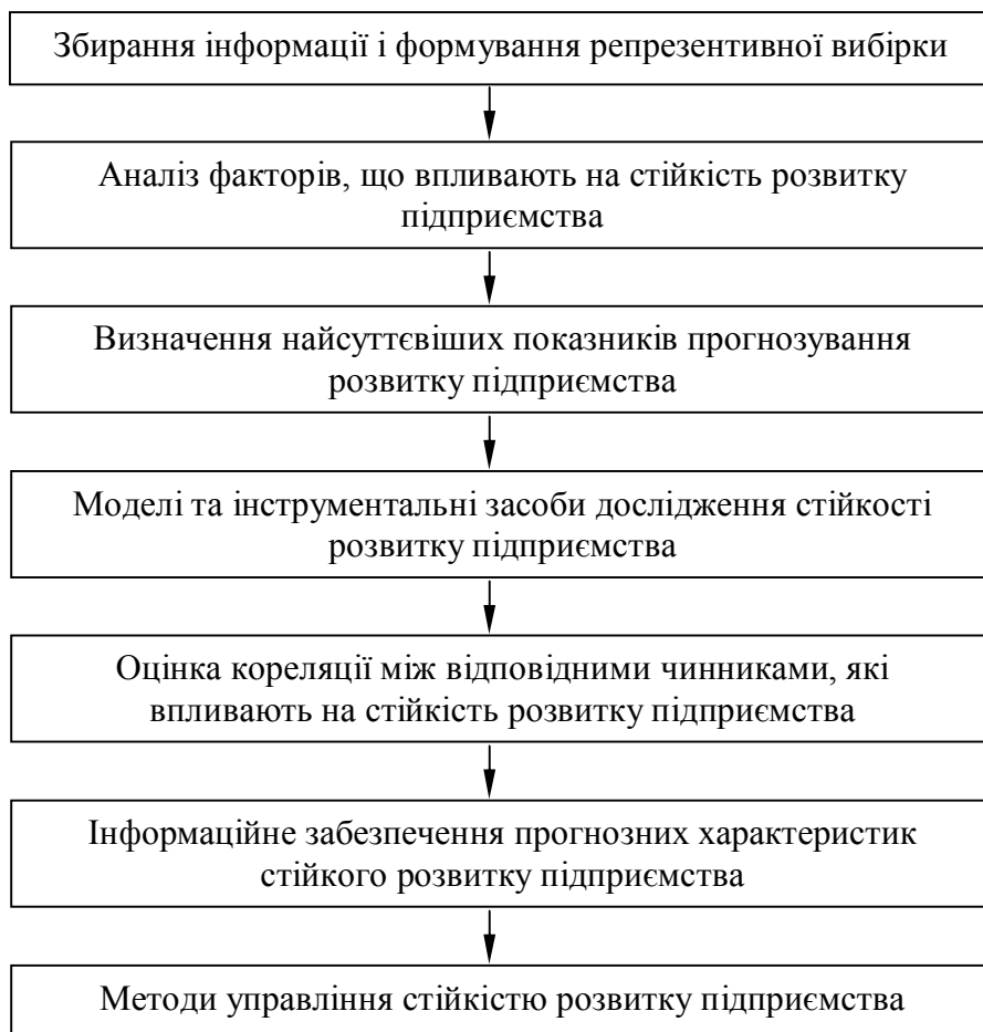
Рис.1 Алгоритм дослідження стійкості розвитку підприємства
