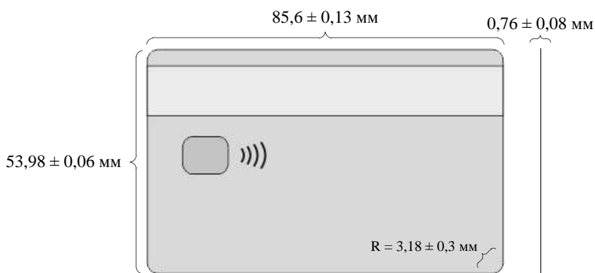
Рис. 5.1 – Фізичні розміри банківської картки (ID-1)
